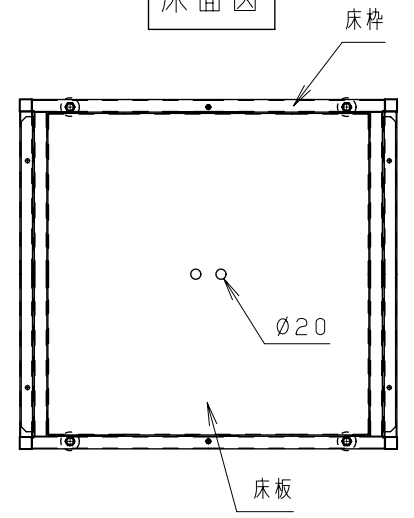
床面図
