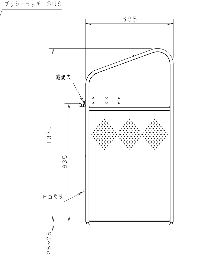
側面図
